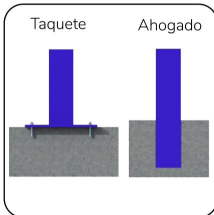
FIJACIÓN DE POSTES
